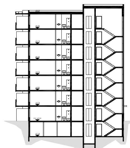
skurður A-A TÝPA 41-43
