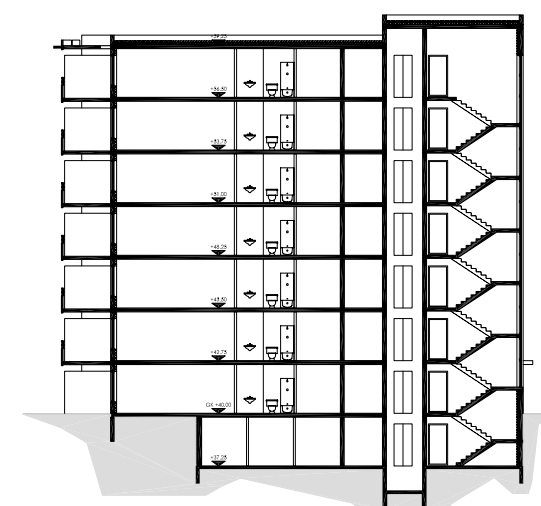
skurður A'-A' TÝPA 45
